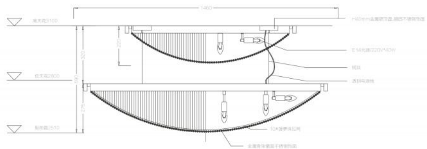
主视图 / Main View
