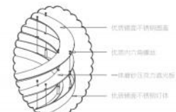
C区局部放大图
