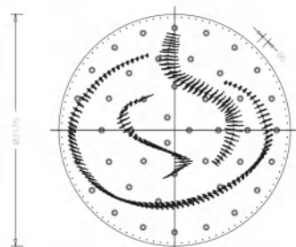
底部视图 / Bottom View
