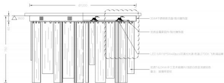
主视图/Front View
