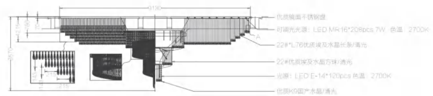
主视图/Front View
