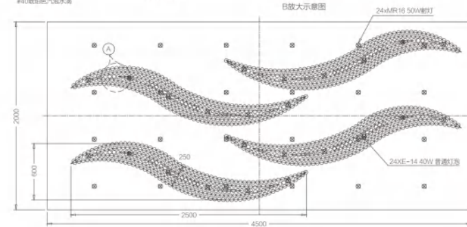
底视图 / Bottom View
