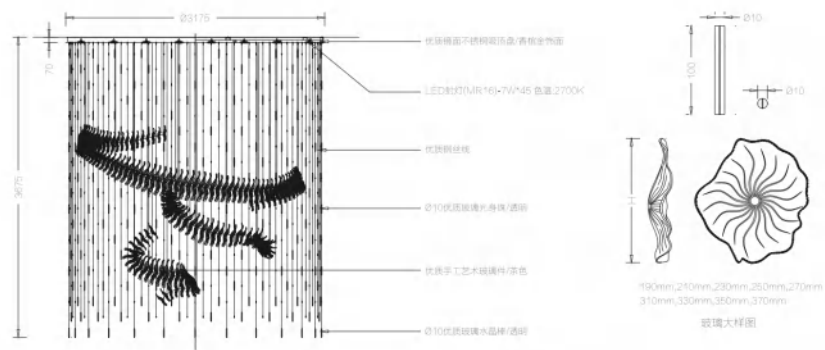
主视图 / Front View
