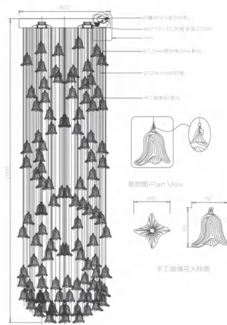
主视图/Front View
