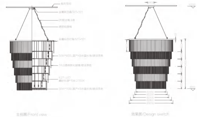
主视图/Front view
